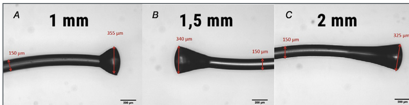
Figura 10 - Forma del bottone di IOL con aptiche in PMMA in base alla distanza con cui viene impugnata l'aptica. (7).
